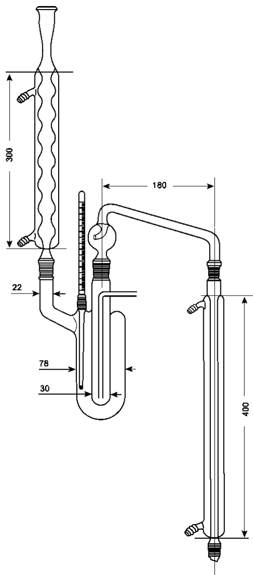
Рисунок 1 – Прибор для определения примесей фторидов Размеры приведены в миллиметрах
